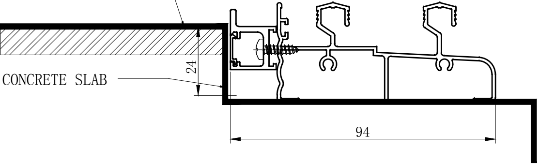
SLIDING DOOR DETAILS
